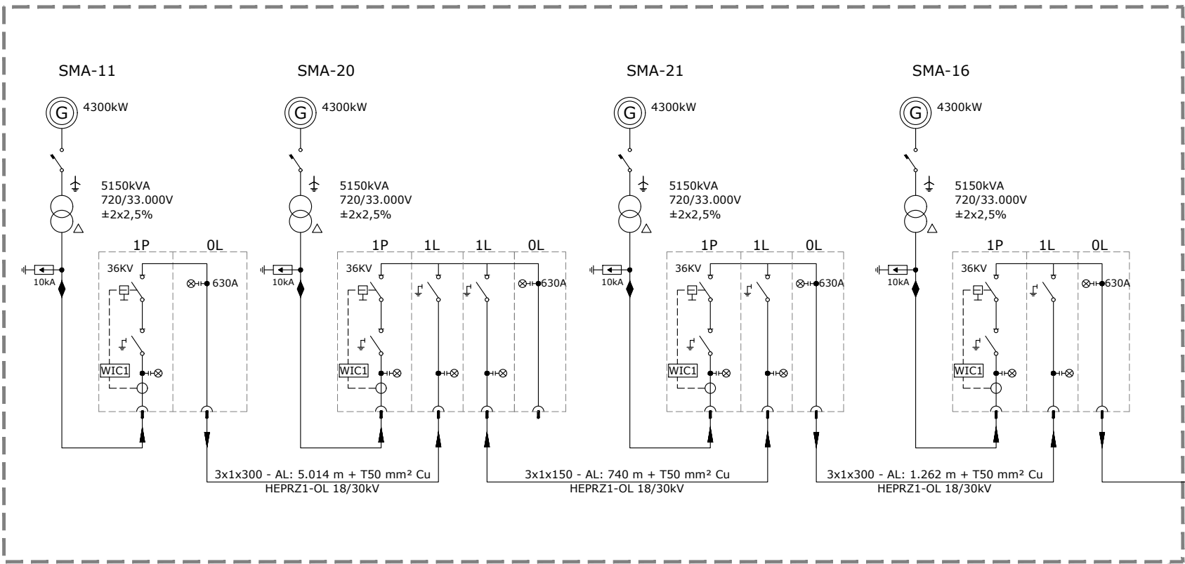
P.E. SAN MATÍAS. CIRCUITO 4
