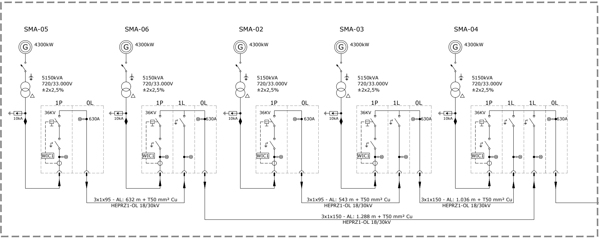
P.E. SAN MATÍAS. CIRCUITO 2
