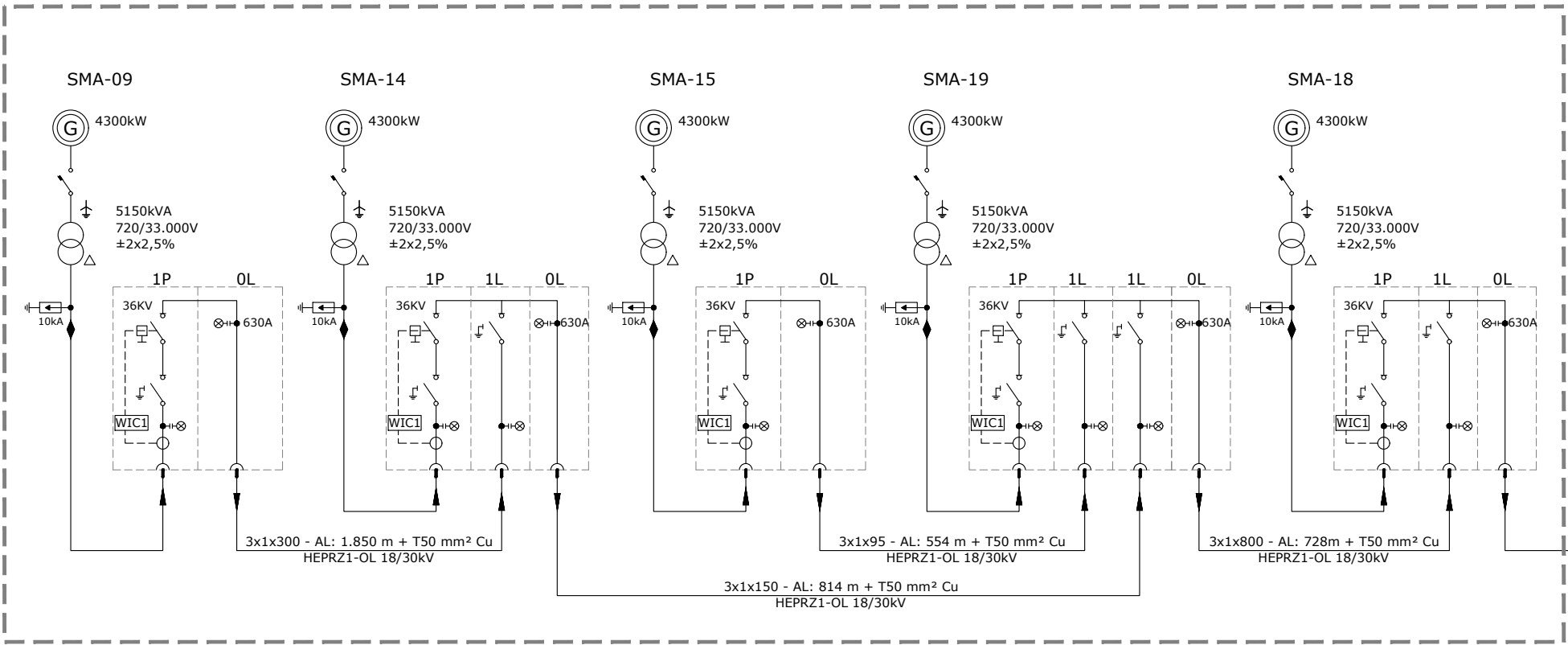
P.E. SAN MATÍAS. CIRCUITO 3
