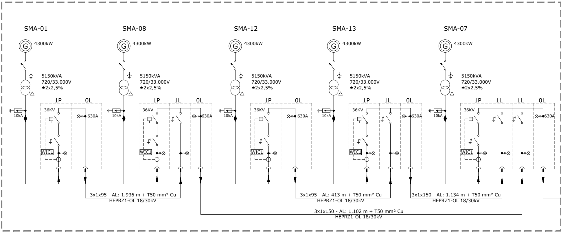
P.E. SAN MATÍAS. CIRCUITO 1
